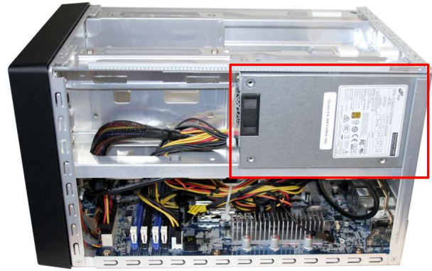
Verwendung des Netzteils FSP500 in einem Shuttle XPC cube SH570R8
